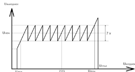
Рисунок 1. Общая диаграмма работы стабилизатора
